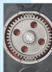
DETALHE CAIXA LATERAL COM ENGENHAGENS
